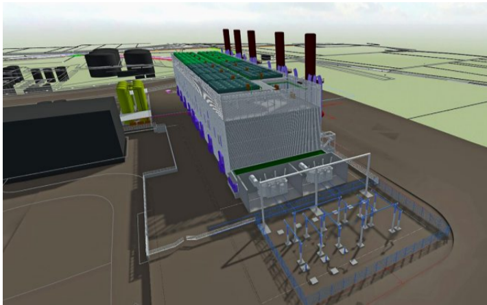
Soll der Schweiz den Strom sichern: Skizze des Reservekraftwerks in Eiken (AG). Bild: zvg
